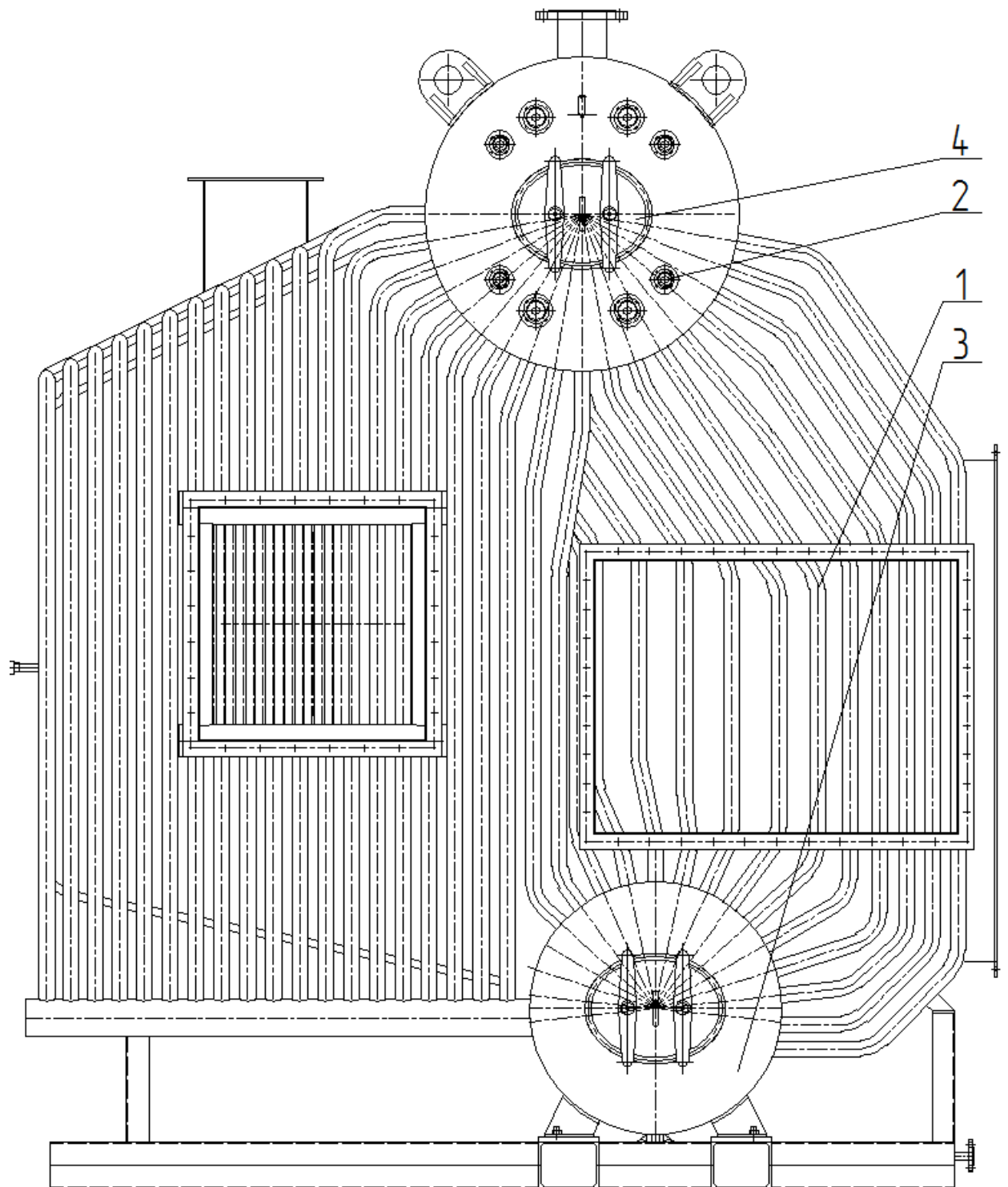
Рис. 2 Система трубная.
